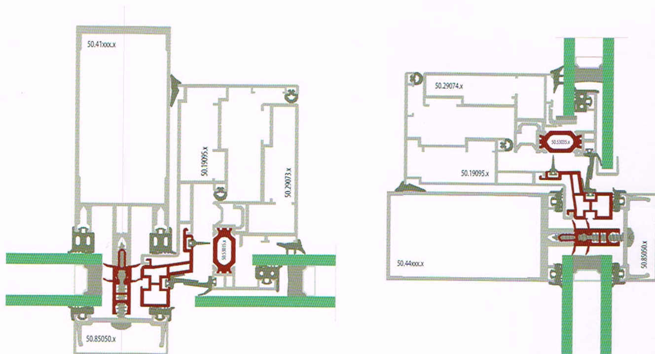
Przekrój przez słup.
