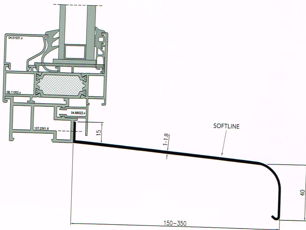
Przekrój przez okno z parapetem typu Softline
