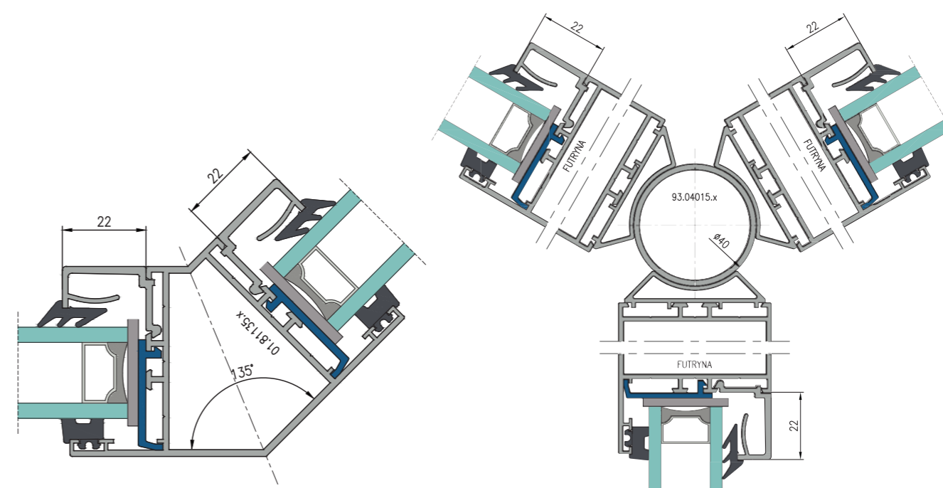
Profil narożny 135°.
