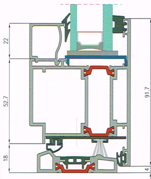
Drzwi progowe ze szczotką.
